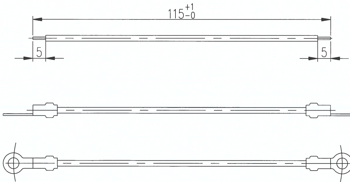
Obr.4 Propojovací kabely P/N:300-753 - výroba
