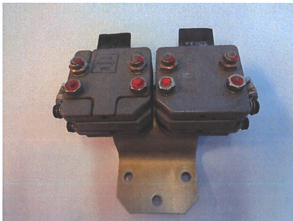
Obr.1 Sestava sběrače P/N:066-5300
