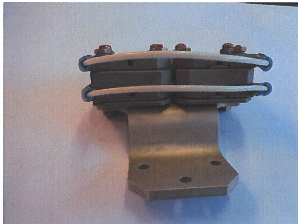
Obr.7 Sestava sběrače P/N:066-5300 s propojovacími kabely P/N:300-753
