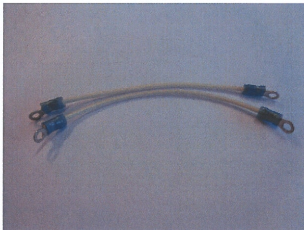
Obr.3 Propojovací kabely P/N:300-753
