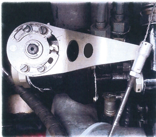
Regulátor LUN7810.( ) Páka ovládání P/N Z43.7800.10.00
